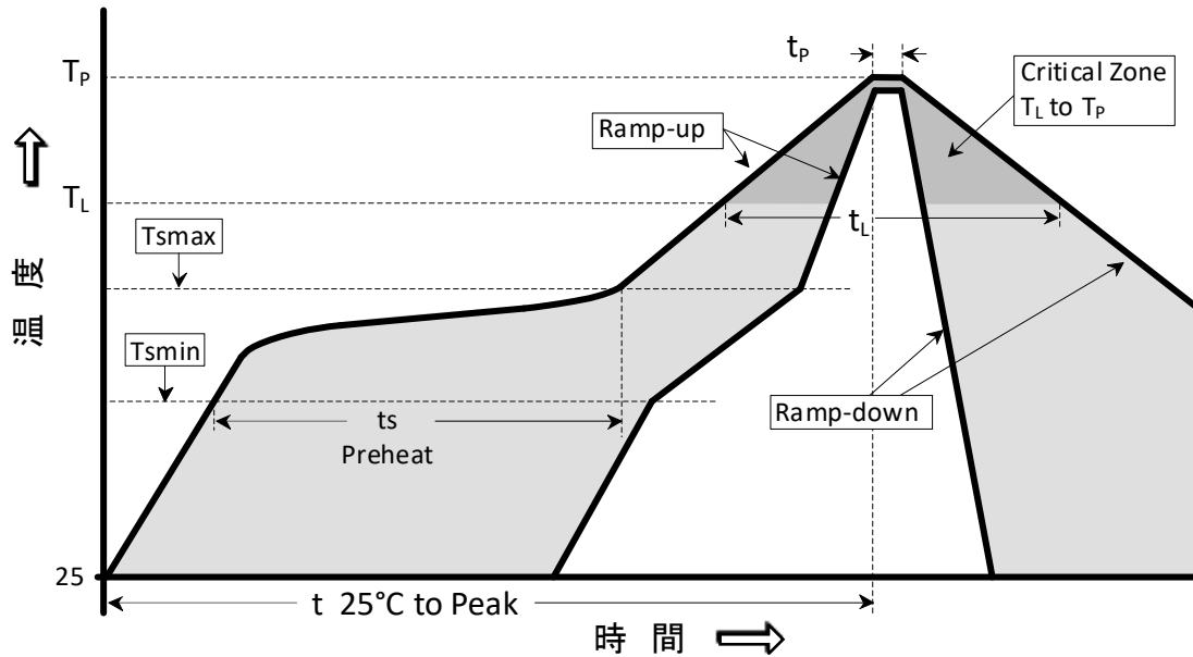
IPC/JEDEC J-STD-020C Pb-free規格 に基づくはんだリフロー条件
