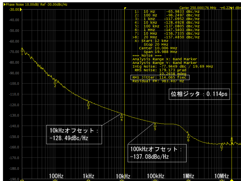
＜ PP224BB-250.000MHz ＞ 位相ノイズ実測例
