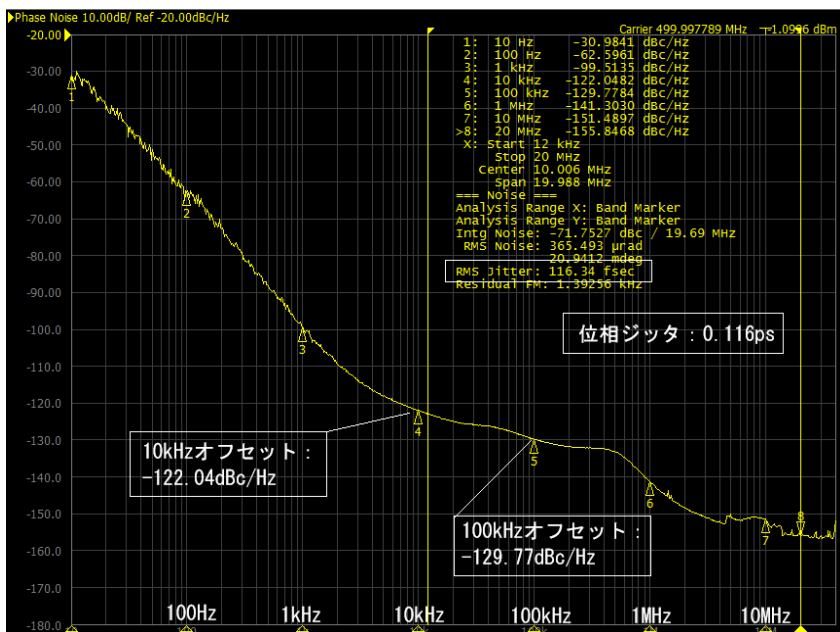
＜ PP224BB-500.000MHz ＞ 位相ノイズ実測例
